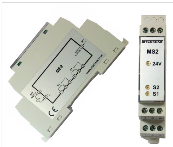
Rys.1 Układ MS2.
