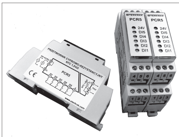
Rys.1 Układ PCR5.
